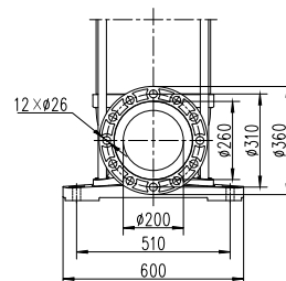
*Фланец PN25/DN200
