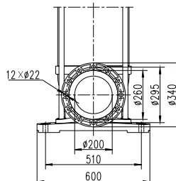
*Фланец PN16/DN200
