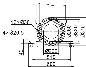
Фланец PN40/DN200
