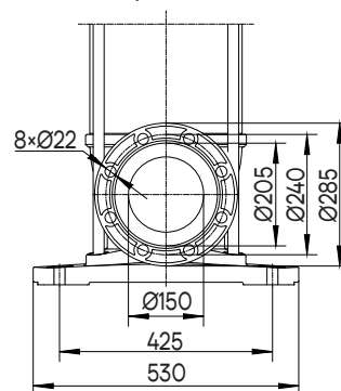
*Фланец PN16/DN150
